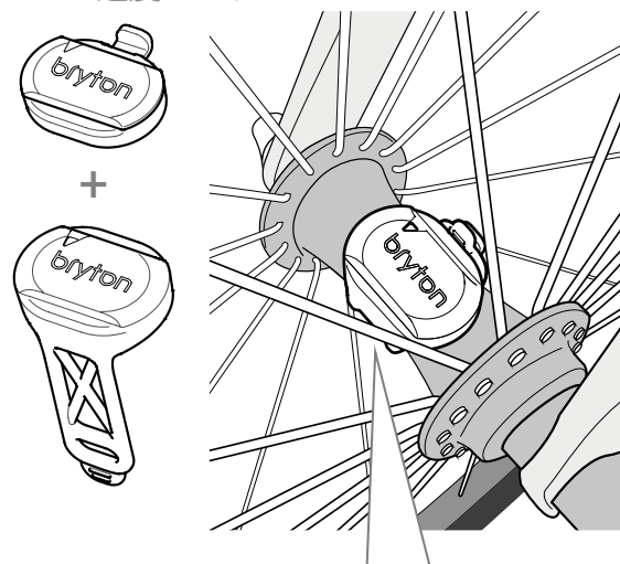
速度センサー
